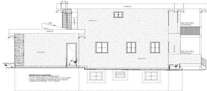
2 Right Elevation
